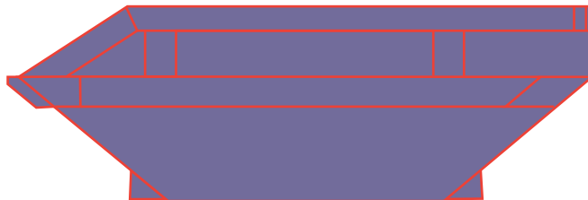
Allzweckmulde 12m 3 4,45 x 2,06 x 1,55
